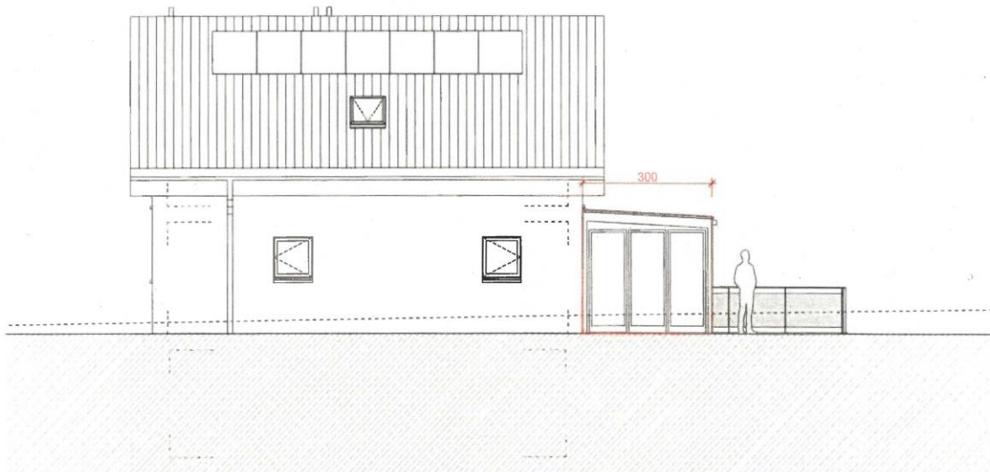
Elévation ouest
