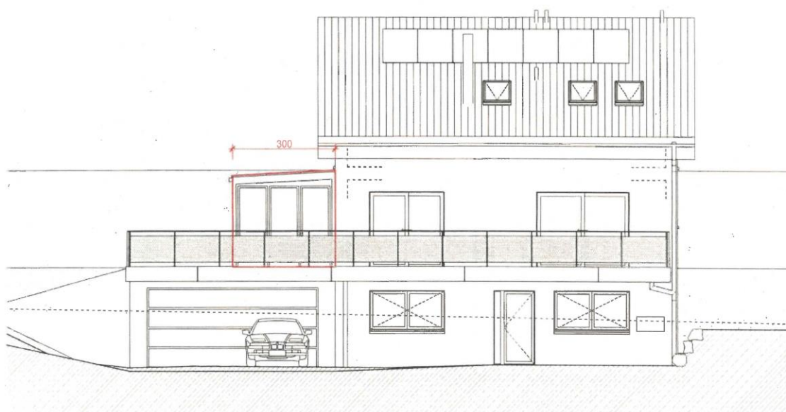
Elévation est
