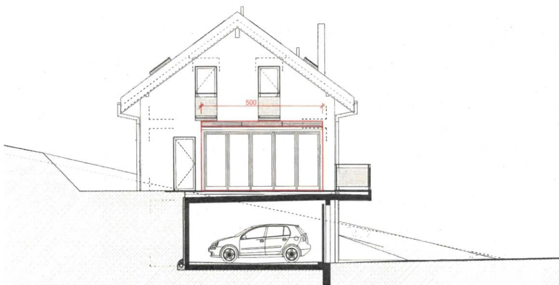
Elévation sud
